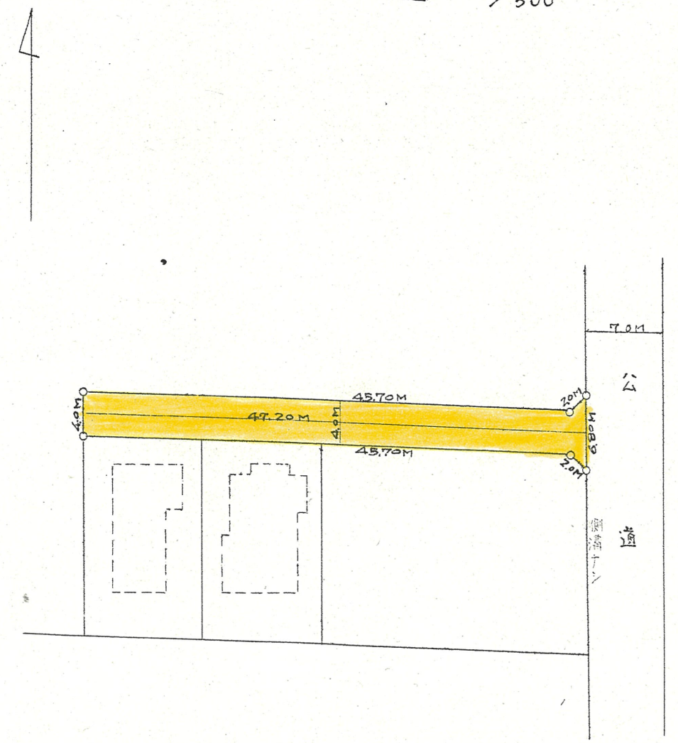
実測図 1/500
