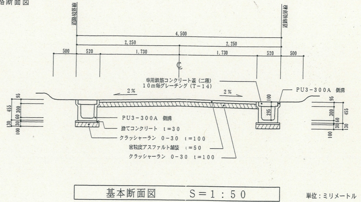
道路断面図
